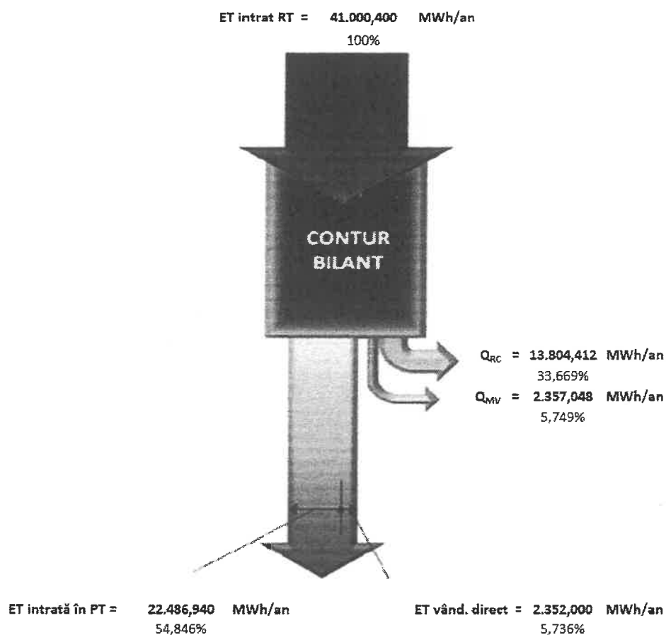
Figura 1 – Diagrama Sankey regim real rețea de transport
