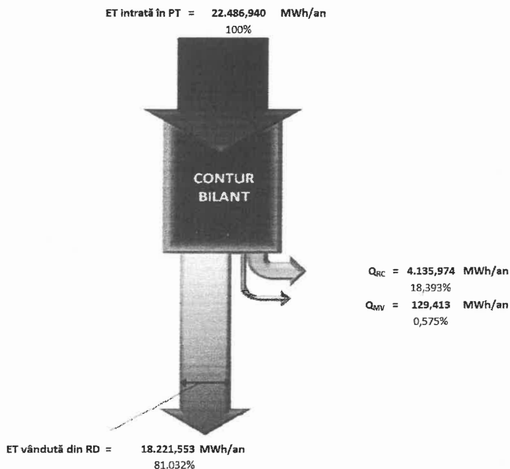
Figura 2 – Diagrama Sankey regim real RD
